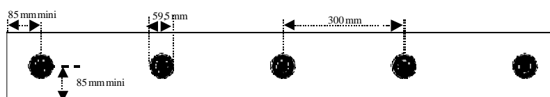
FIGURE 8: CIBLERIE VITESSE 5 CIBLES
